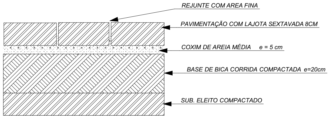
DETALHE 01/CORTE - PAVIMENTAÇÃO sem escala
