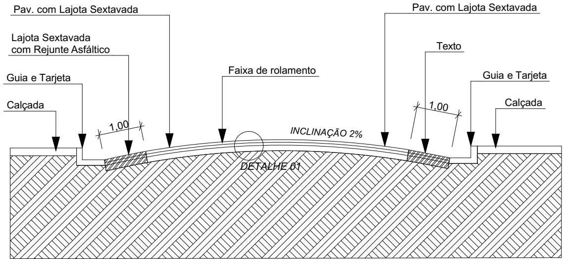
Seção Transversal das vias sem escala
