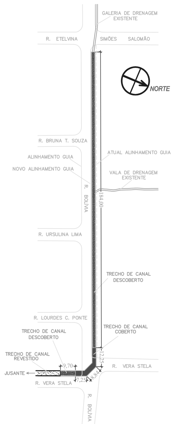
PLANTA DO CANAL 2 - TRECHO RUA BOLÍVIA ESC. 1:500
