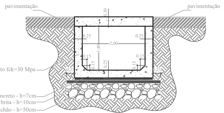
SEÇÃO DO CANAL - COBERTO ESC. 1:20
