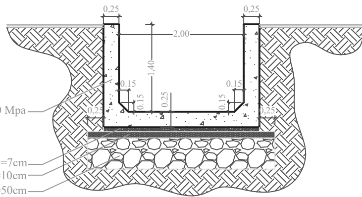
SEÇÃO DO CANAL - DESCOBERTO ESC. 1:20
