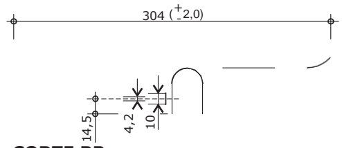
CORTE BB ESC. 1:5
