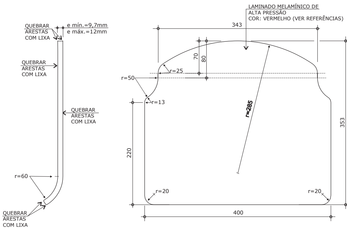
VISTA LATERAL
