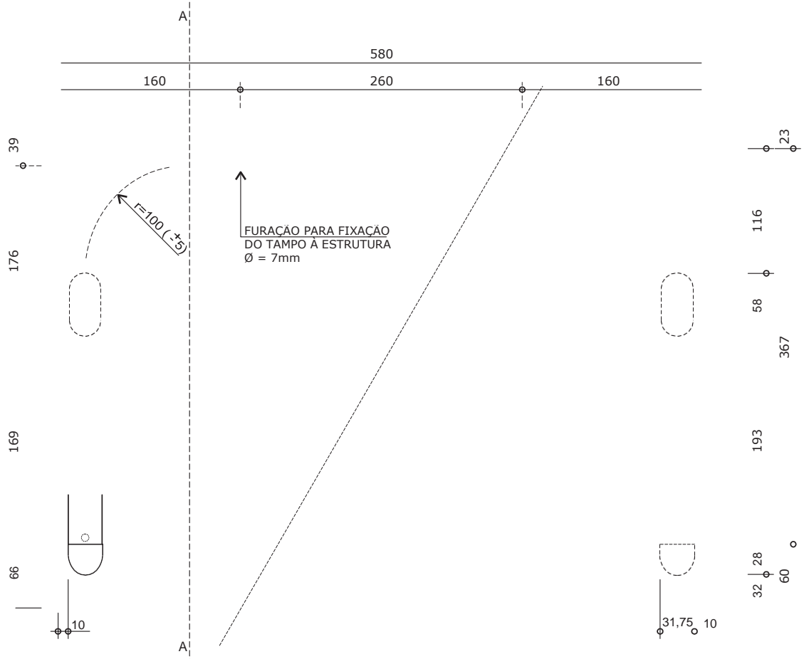
VISTA SUPERIOR
