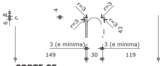
CORTE CC ESC. 1:5
