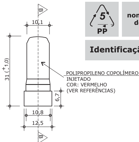
VISTA 3 ESC. 1:1
