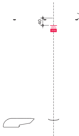
ETIQUETA CENTRALIZADA EM RELAÇÃO AO TUBO
