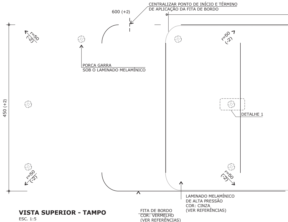
VISTA SUPERIOR
