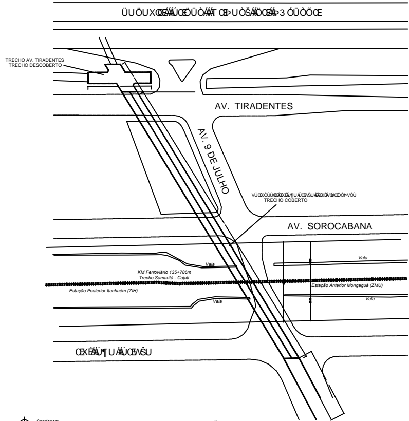
02 PLANTA DE IMPLANTAÇÃO ESC 1:500
