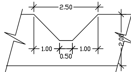
DETALHE DAS VALAS - SEÇÃO ESC. 1:50
